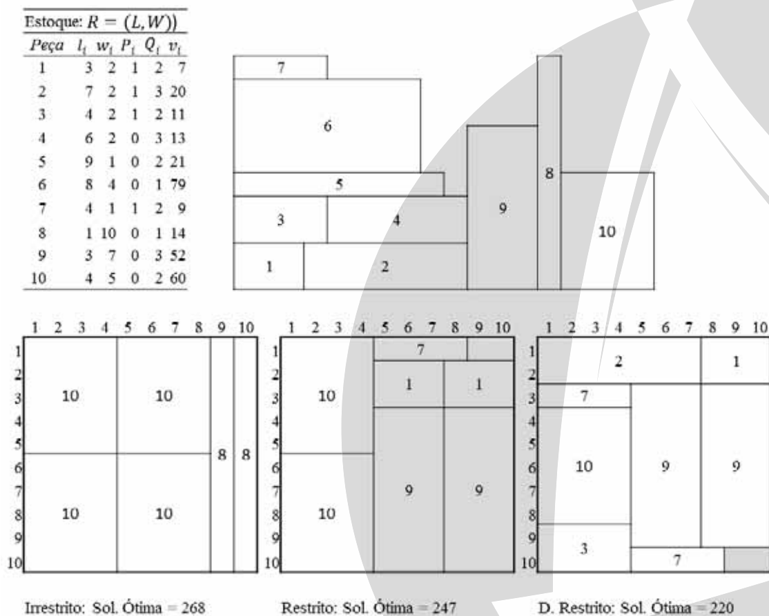
Figura 1 – Exemplo de solução para o problema de corte. Adaptado de Alvarez-Valdes et al. (2007).
