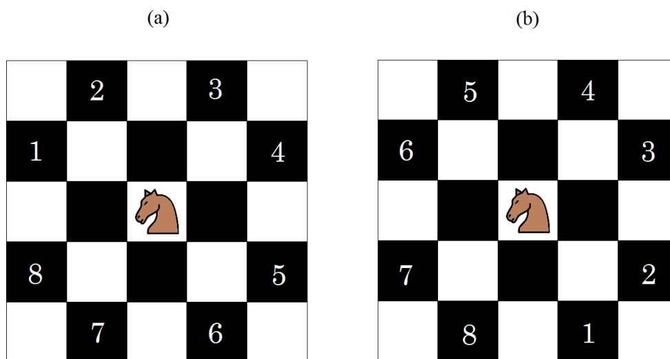
Figura 4. Permutações das prioridades: (a) casa inicial no primeiro octante; (b) casa inicial no sexto octante.
